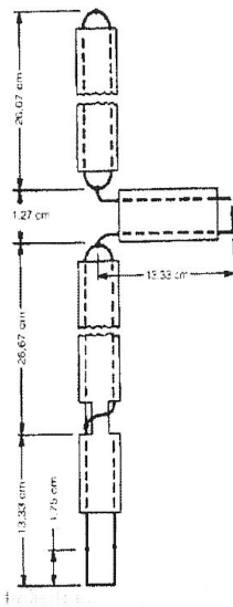
Figure 2. Schéma électrique de la colinéaire à deux éléments.
