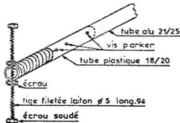
Fig. 2. — Détail self et tige d'accord.
