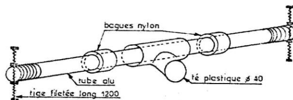
Fig. 5. — Élément réflecteur. Les bagues nylon maintiennent le tube à l'intérieur du té plastique.
