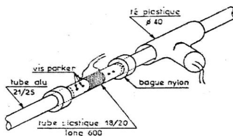
Fig. 3. — Attaque du radiateur. Le té plastique vient recouvrir les bagues nylon.
