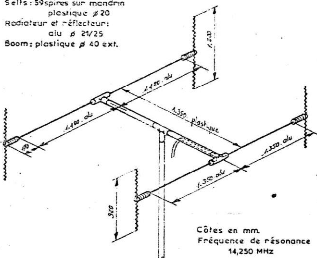
Fig. 1. — Vue d'ensemble de l'antenne.
